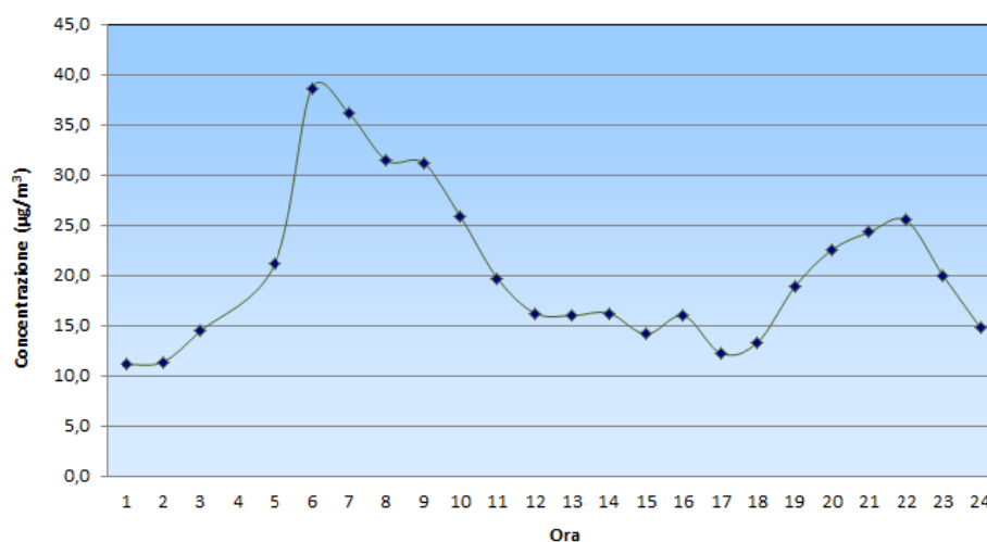
SITO RICETTIVO "MOLINARI" - DAL 07/06/2016 AL 06/07/2016 Biossido di azoto: giorno tipo
